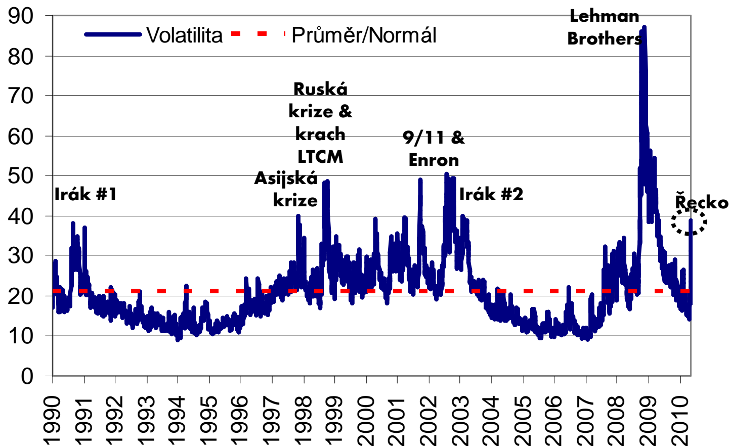
VOX/VIX INDEX - volatilita/proměnlivost/kolísání hlavního amerického akciového indexu S&P 500
